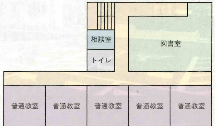
2階平面図
