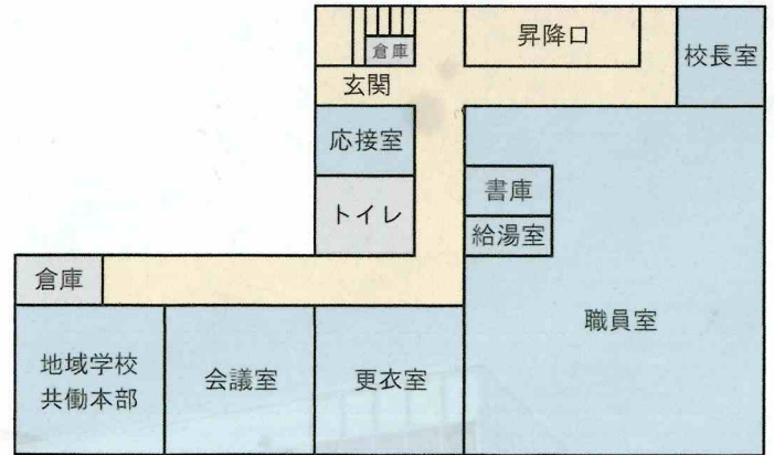
1階平面図
