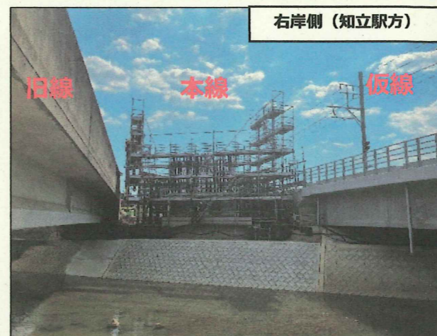
逢妻男川渡河部（上流より下流側を望む）
